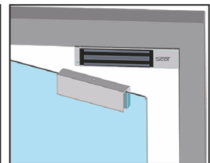
Montaż z uchwytem BK-800UL
